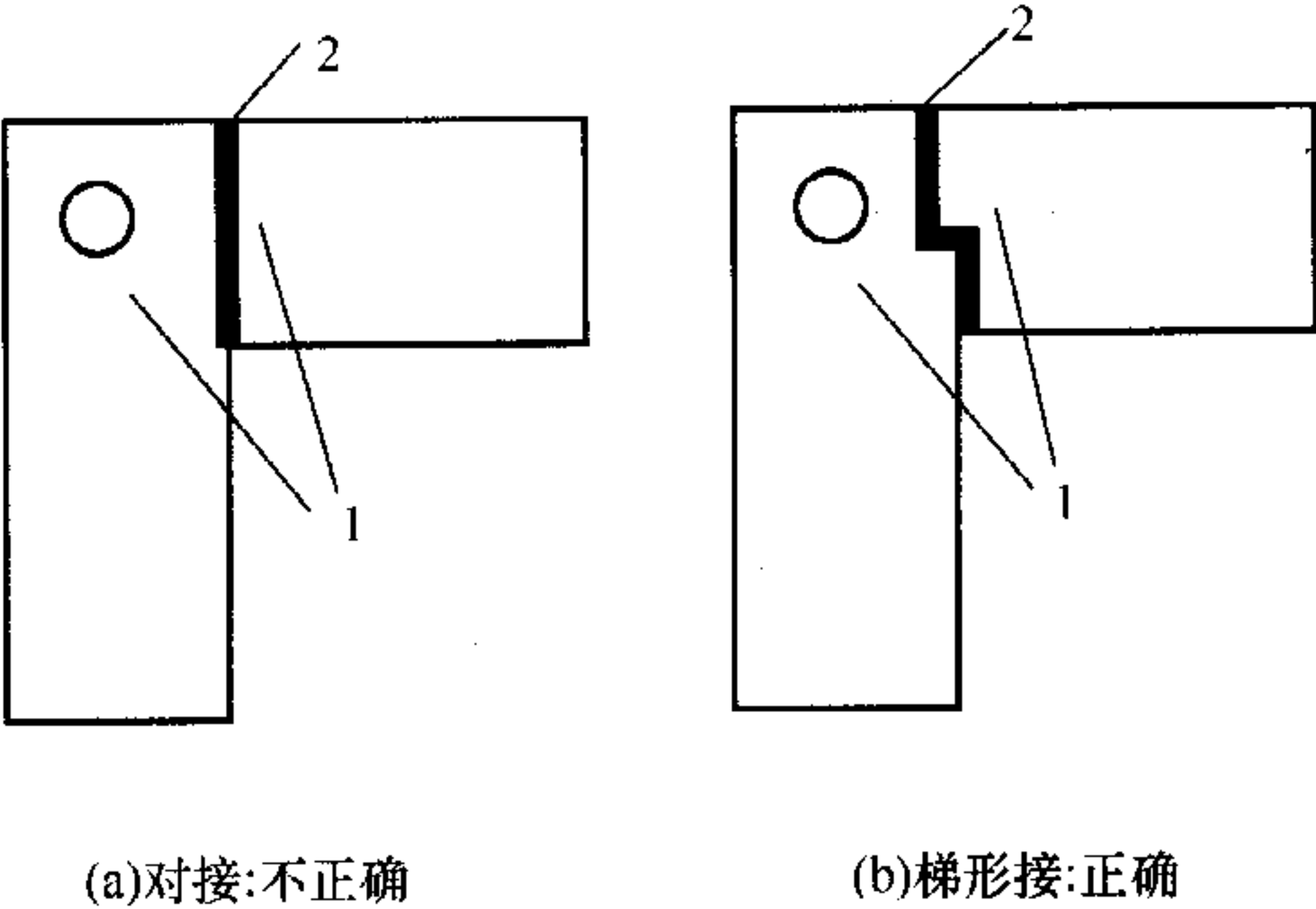
图 5.3.3 法兰密封垫接头 1—密封垫；2—密封胶
