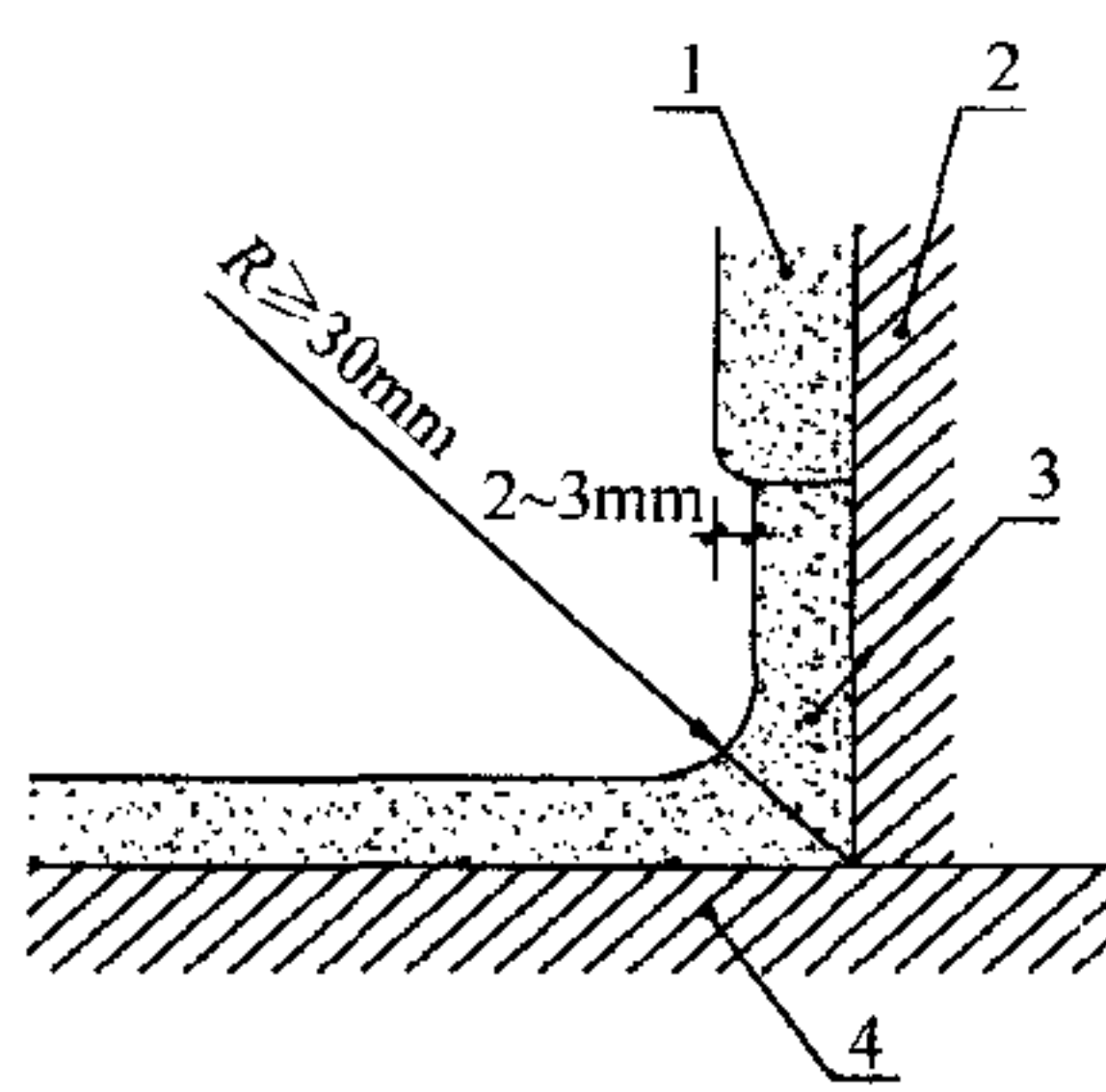
图 4.5.1 整体墙角的圆弧做法 1—墙体；2—墙体基层； 3—整体墙角；4—地面
