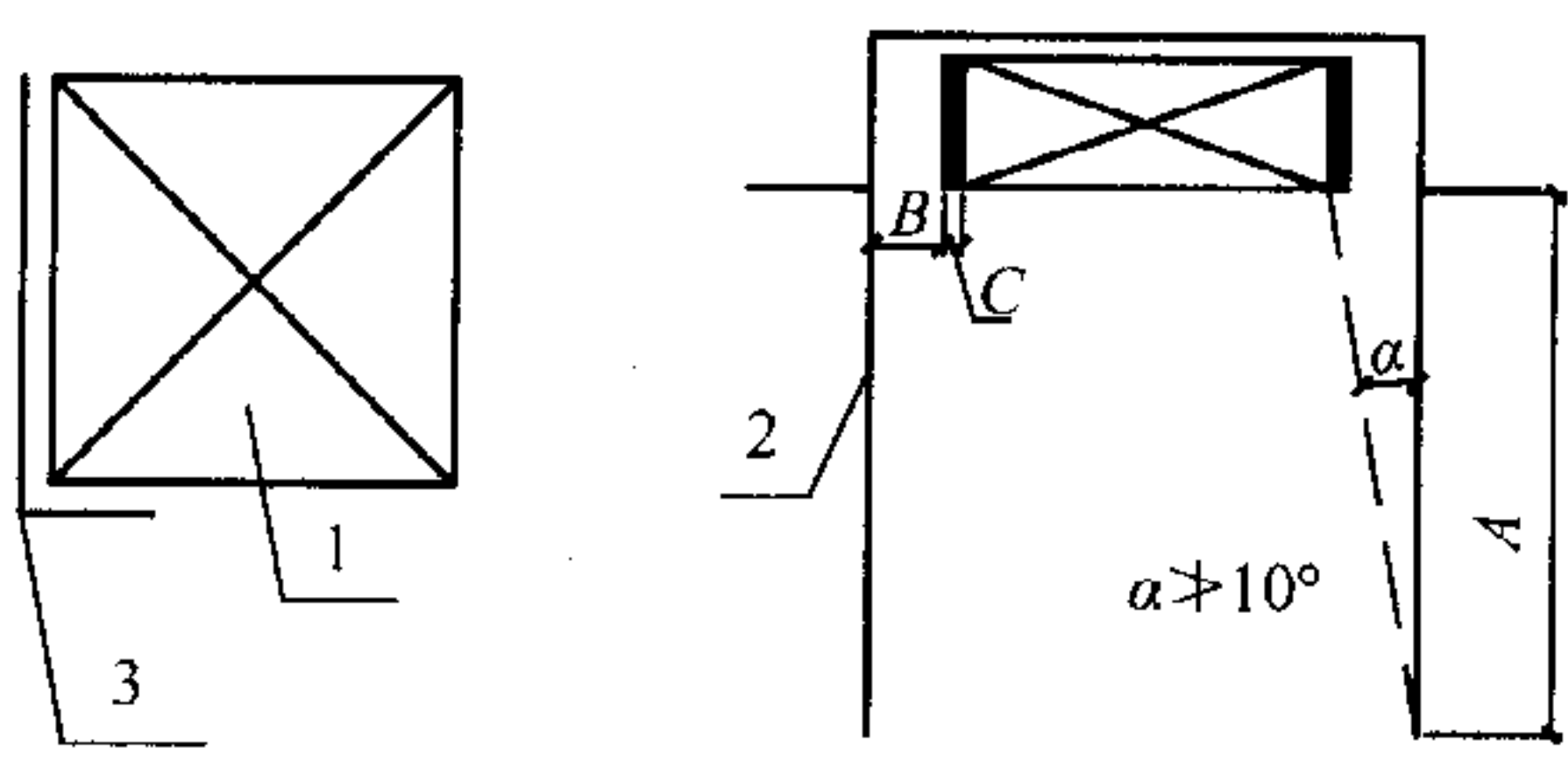
图 D. 3. 10 检漏用挡板或围挡管
