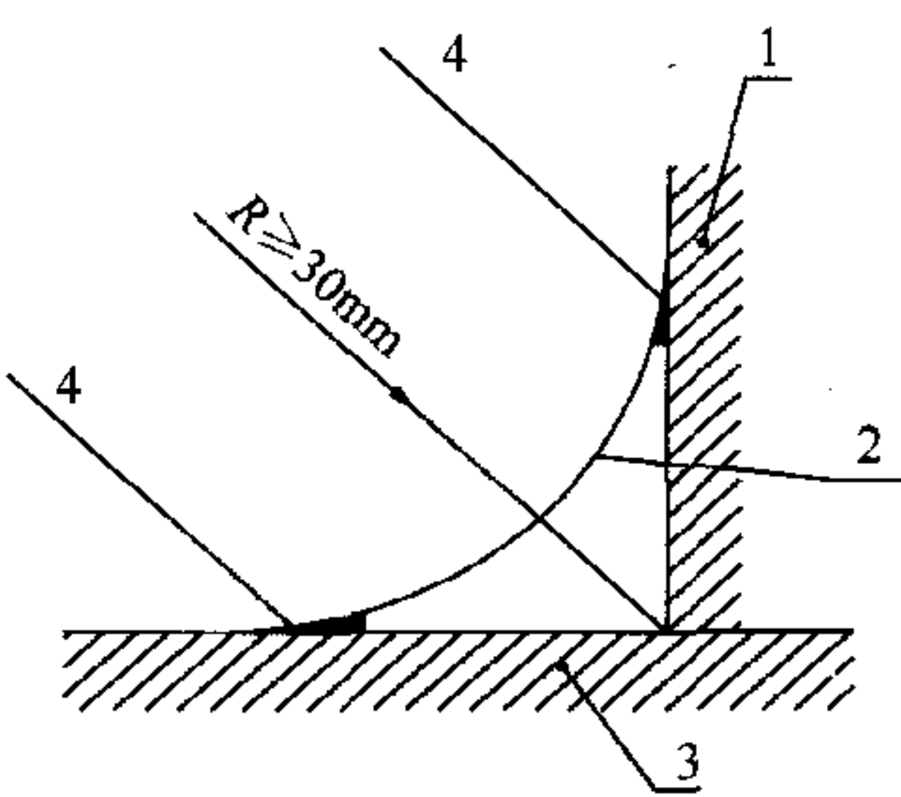
图 4.5.2 型材过渡墙角的圆弧做法 1—墙体；2—型材墙角； 3—地面；4—密封嵌固材料
