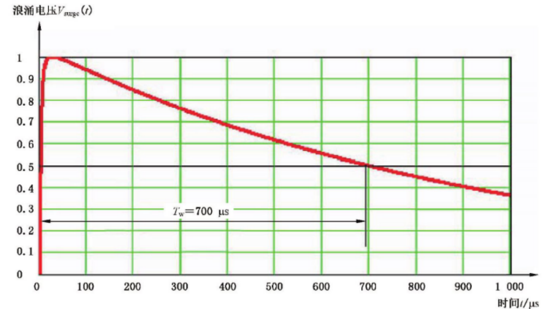
图 E.7 浪涌电压(10/700 \mu\text{s} ):响应持续时间 T_w
