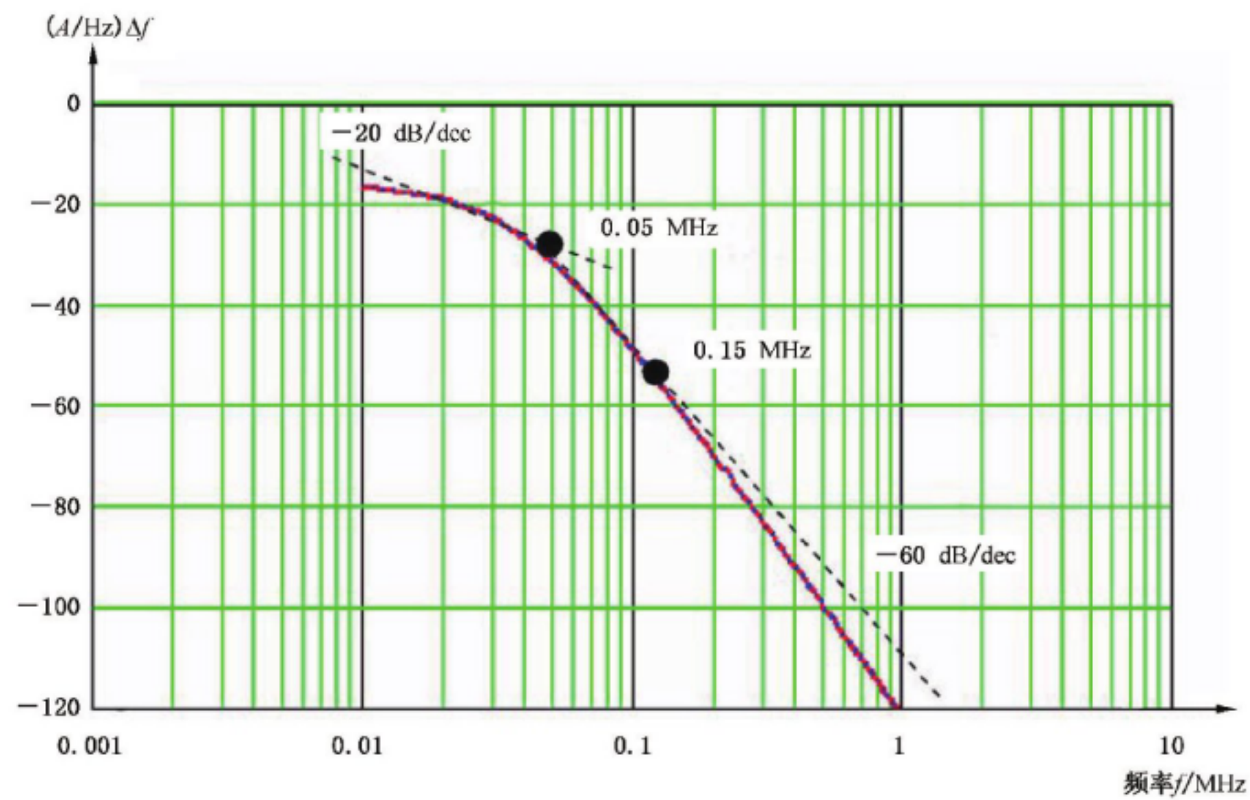
图 E.6 浪涌电流(8/20 \mu\text{s} ):频域响应图, \Delta f = 10 \text{ kHz}
