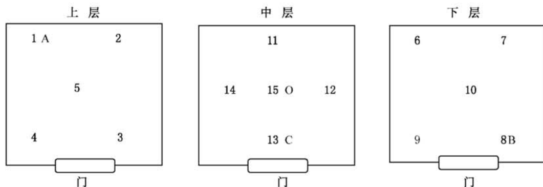
图2 设备容积大于2 m³布点示意图
