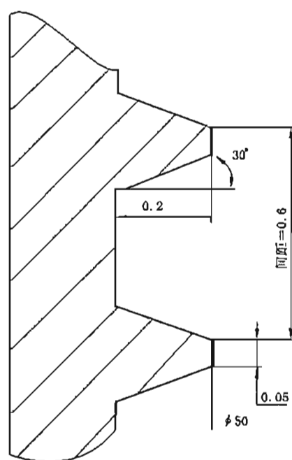
图 111 深腔管局部剖面图(举例)
