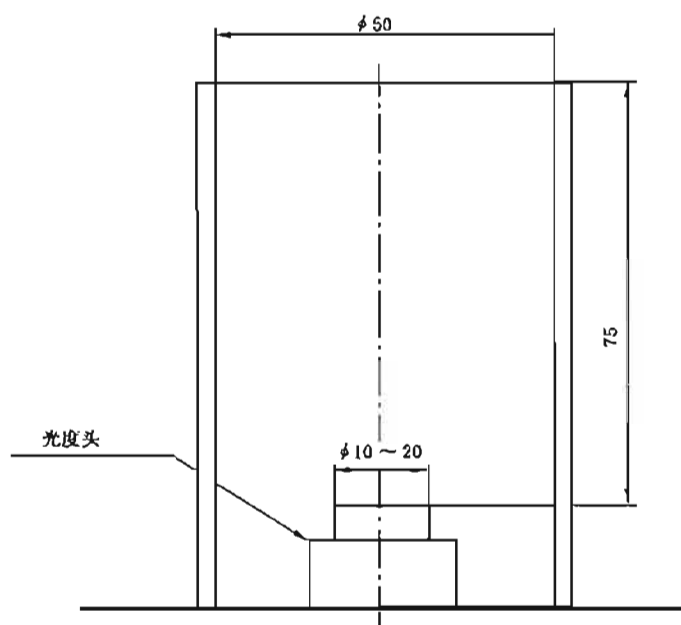
图 110 深腔管底部照度测量
