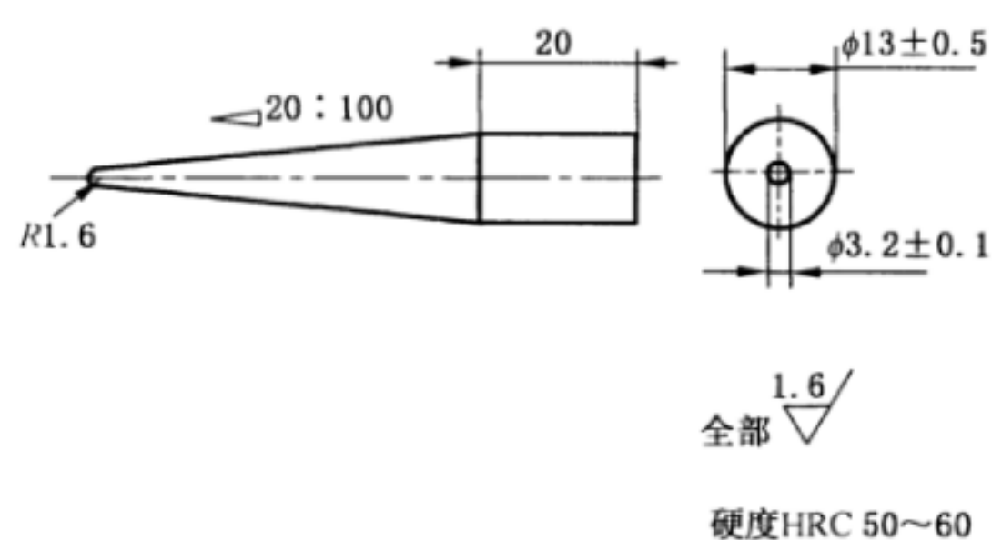
图 1 戳穿试验测头
