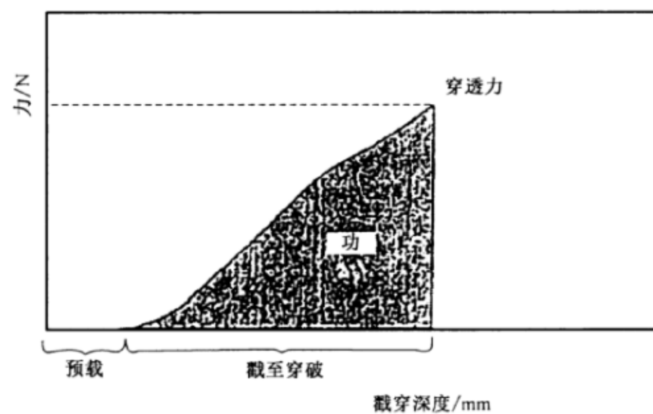
图 3 慢速戳穿试验图示输出
