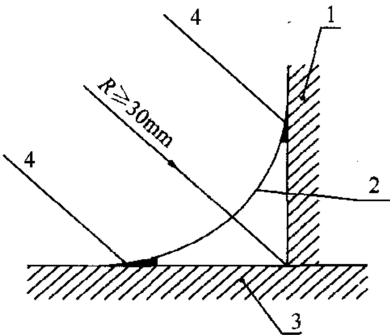
图 4.5.2 型材过渡墙角的圆弧做法 1—墙体；2—型材墙角； 3—地面；4—密封嵌固材料
