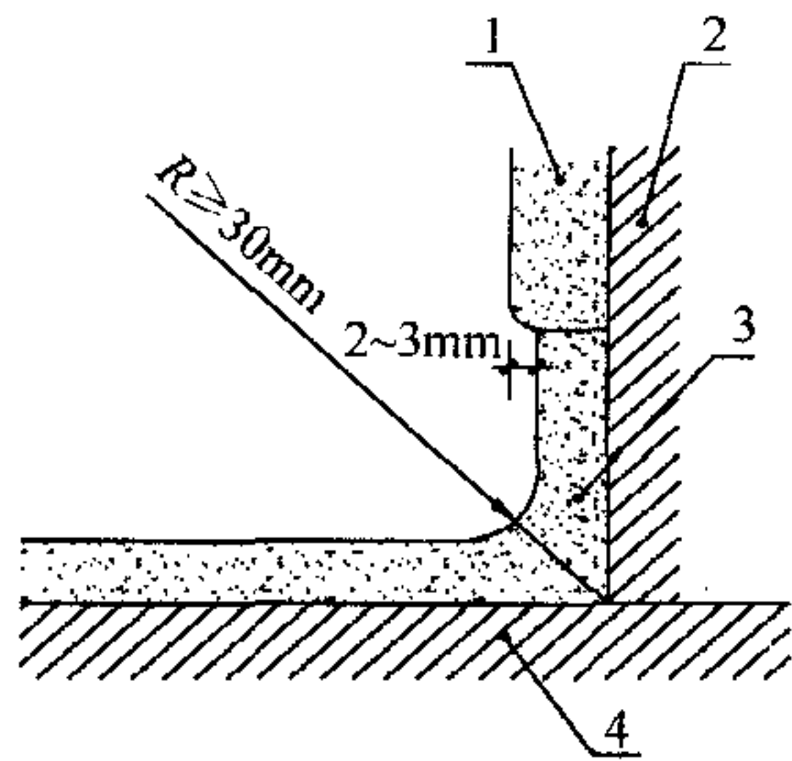
图 4.5.1 整体墙角的圆弧做法 1—墙体；2—墙体基层； 3—整体墙角；4—地面
