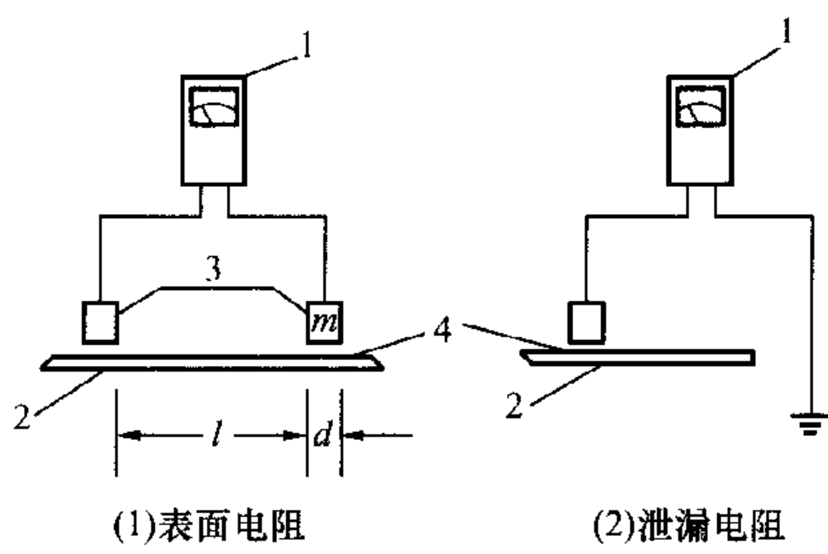
图 E. 9. 3 表面导静电性能测试装置 1—高阻计；2—试件； 3—铜圆柱形电极， m ；4—湿渍纸 l=900\text{mm} ； d=60\text{mm} ； m=2\text{kg}
